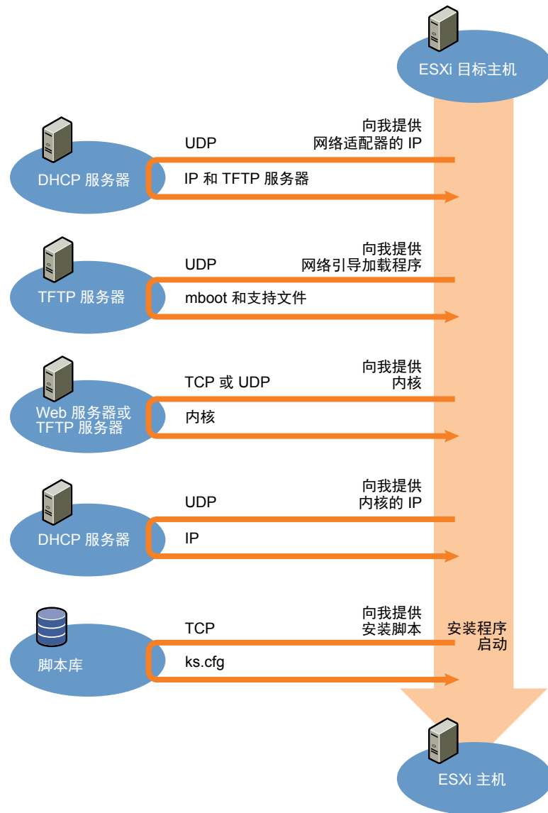
图 3-1. PXE 引导安装过程概览
