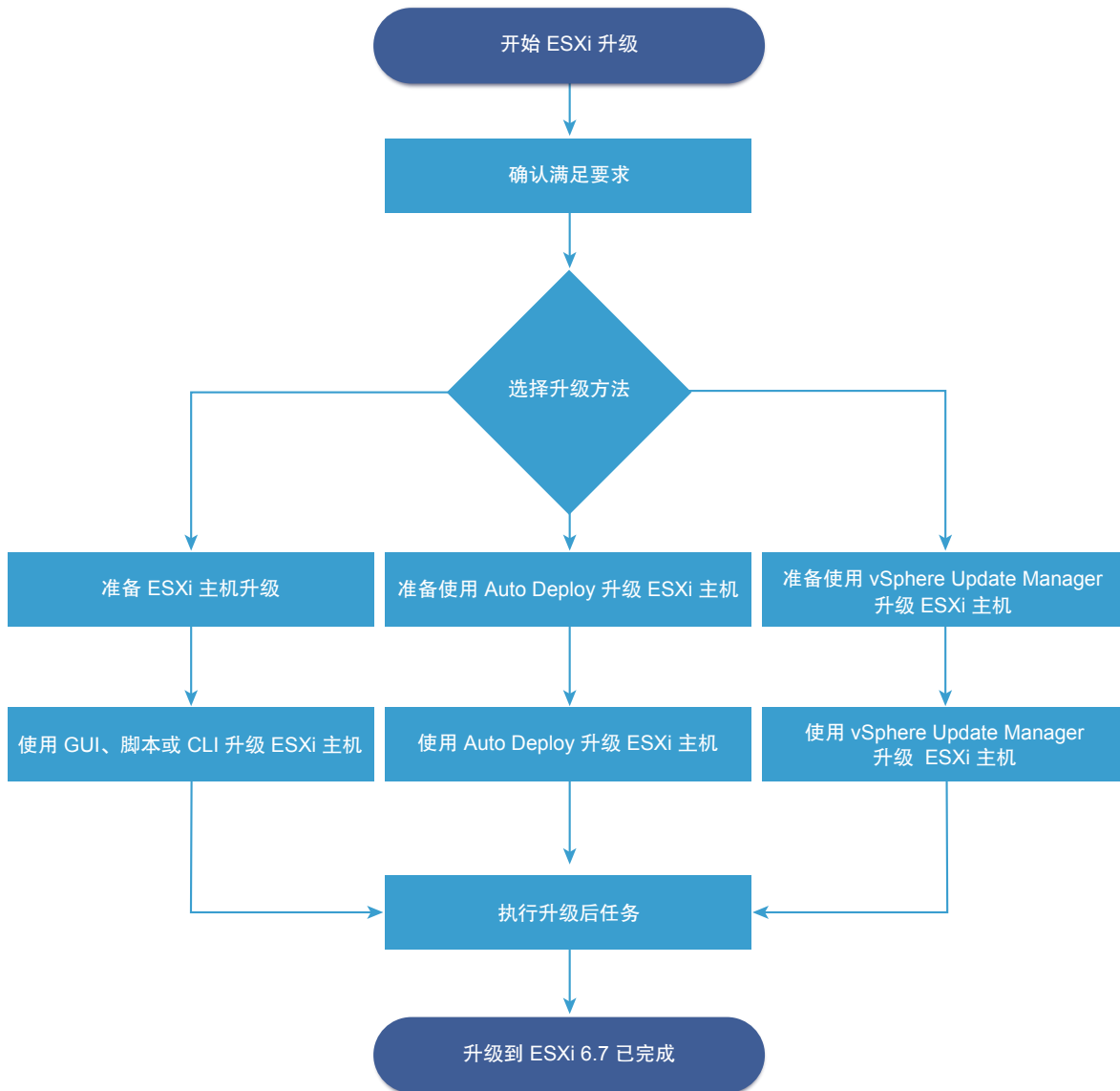
图 2-2. ESXi 主机升级过程概览
